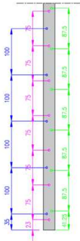
Kuva 20: Kiskojen etupinnan reikäjako
