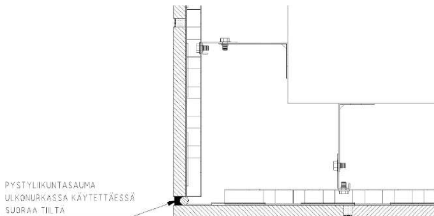
Kuva 44: Pystyliikuntasäuma ulkonurkassa suoralle laatalle
