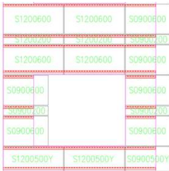
Kuva 23: Asennuskiskot ikkunan ympärillä
