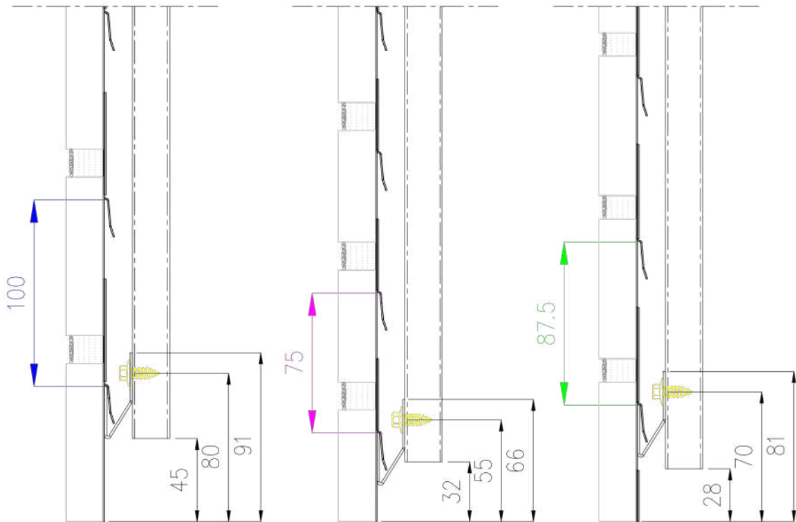
Kuva 17: Verhouksen alareunan mitoitus kylmäverhousjärjestelmälle eri etenemille
