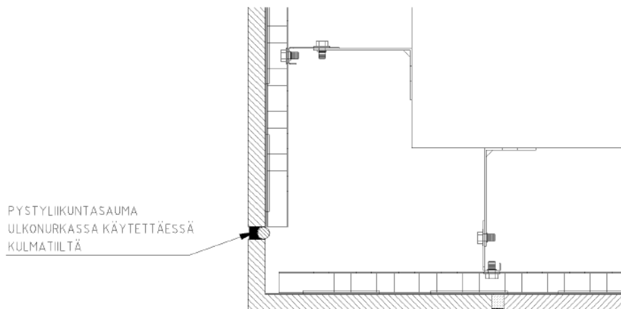
Kuva 45: Pystyliikuntasäuma ulkonurkassa kulmalaatalle
