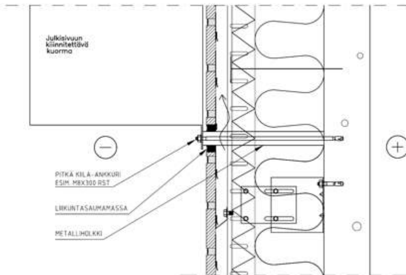
Kuva 39: Ulkoisen kuorman kiinnitys kantavaan rakenteeseen
