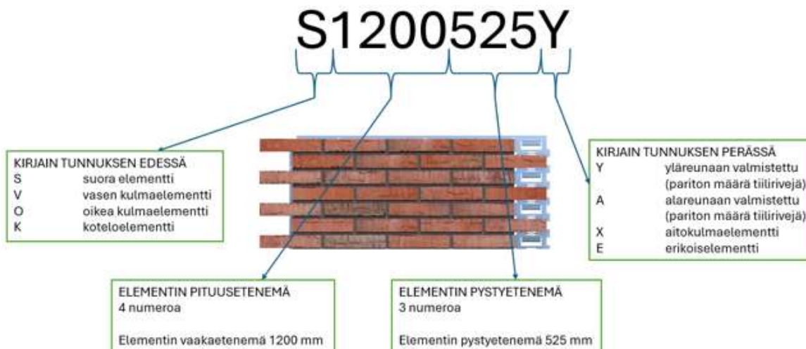
Kuva 3: Tiiliverhouslevyjen tunnukset
