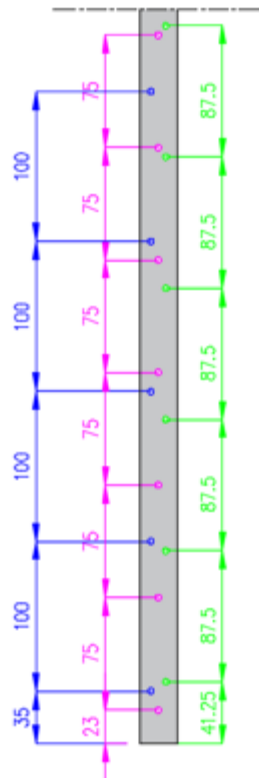
Kuva 20: Kiskojen etupinnan reikäjako
