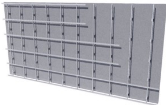
Kuva 25: Asennuskiskojako villinä
