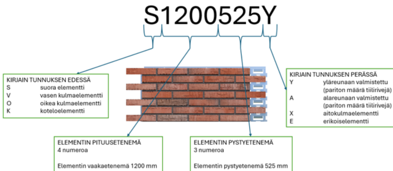
Kuva 3: Tiiliverhouslevyjen tunnukset
