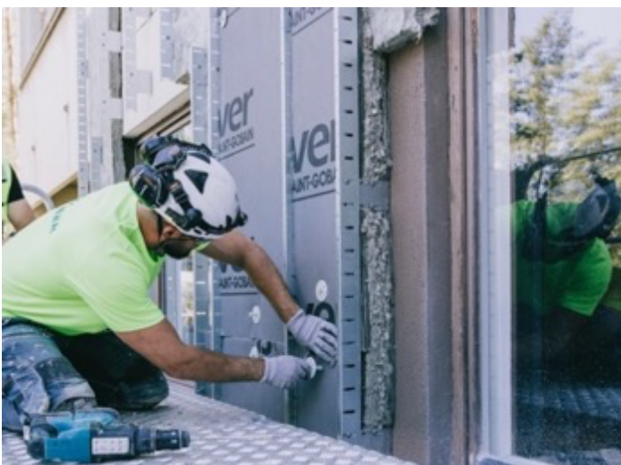
Kuva 32: Tuulensuojaeristyksen asentaminen
