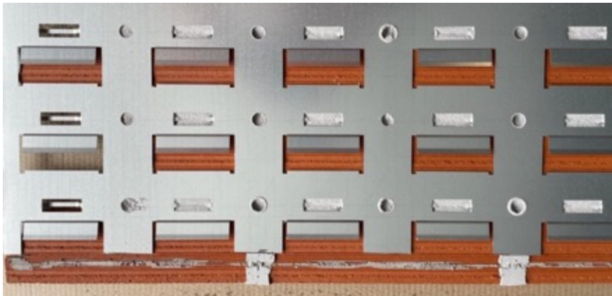
Kuva 33: Runkopelti leikattu alareunan verhouslevyistä
