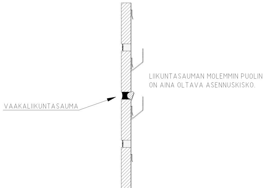
Kuva 43: Leikkauskuva vaakaliikuntasaumasta
