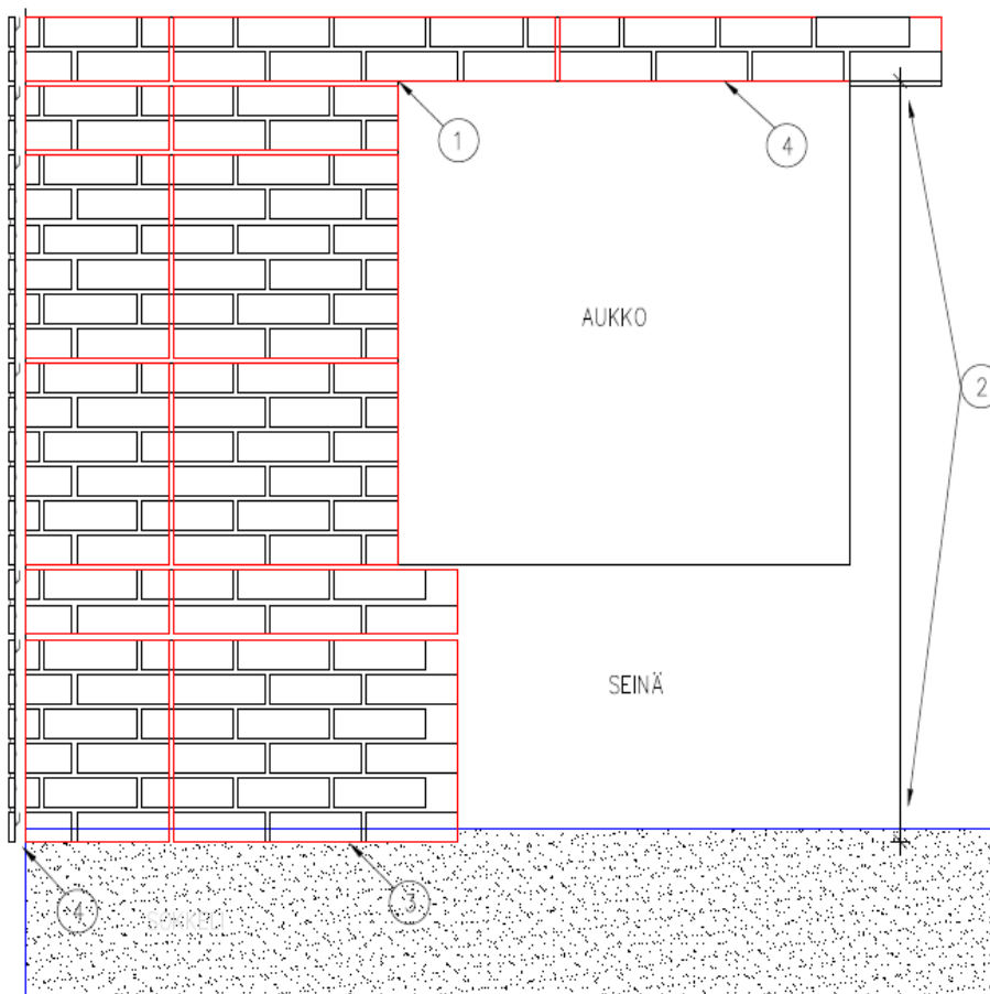
Kuva 16: Tiiliverhouksen alareunan mitoitus
