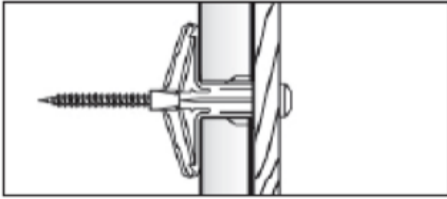
Kuva 38: Kevyen rakenteen kiinnittäminen ohutlevyankkuria apuna käyttäen
