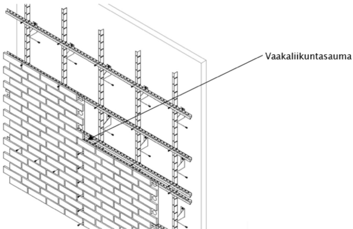
Kuva 42: Vaakaliikuntasauma
