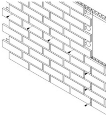
Kuva 35: Poraruuvien paikat tiiliverhouslevyjen liitoskohtiin
