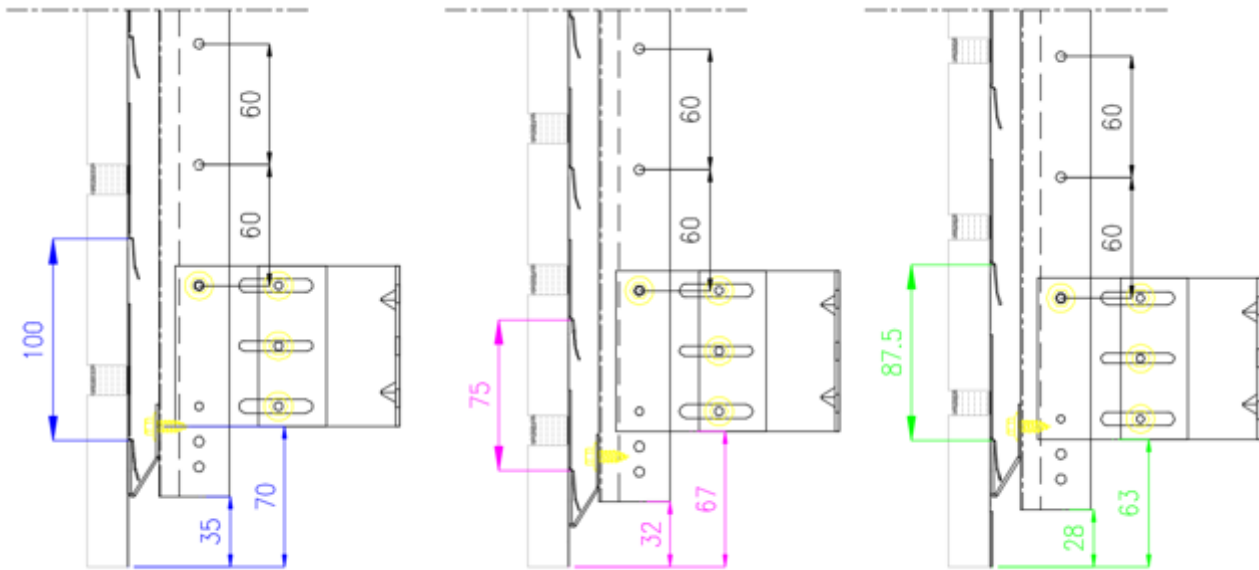
Kuva 27: Seinäkiinnikkeiden asennuskorko tiliverhouksen alareunaan verrattuna
