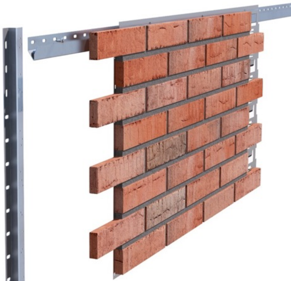
Kuva 14: Kiinnitysjärjestelmä kylmäverhoukselle
