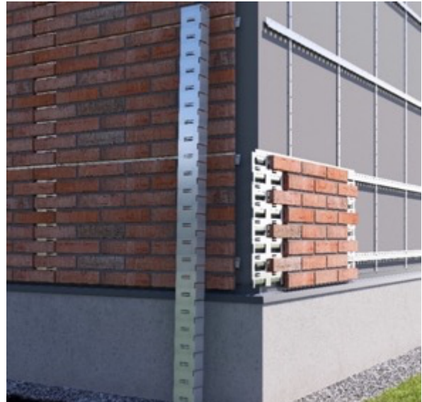
Kuva 4: Kulman valmistaminen työmaalla kulmapeltiin
