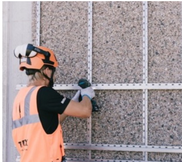
Kuva 24: Asennuskiskojen asennus
