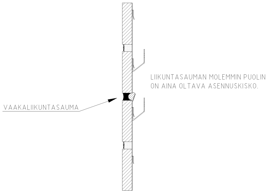
Kuva 43: Leikkauskuva vaakaliikuntasäumasta
