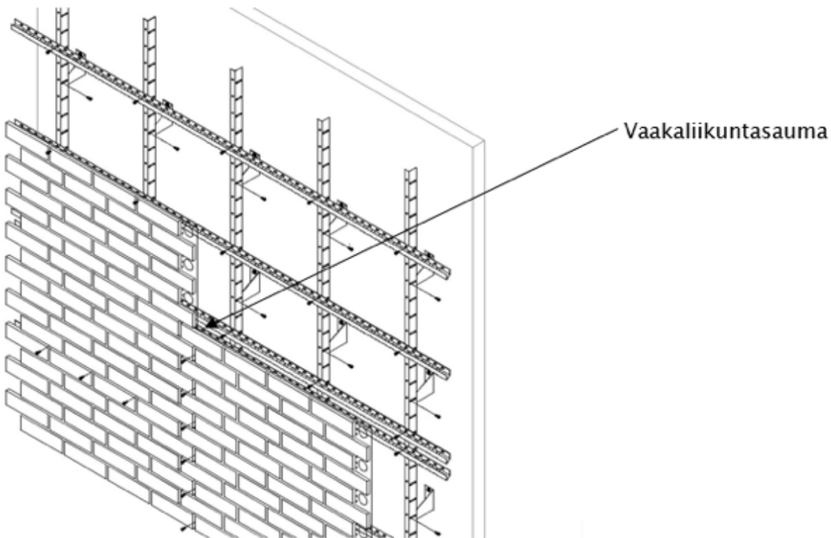
Kuva 42: Vaakaliikuntasauva
