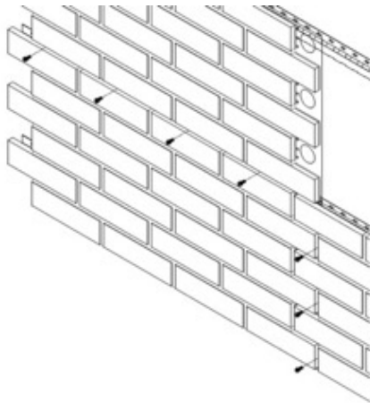
Kuva 35: Poraruuvien paikat tiiliverhouslevyjen liitokohtiin
