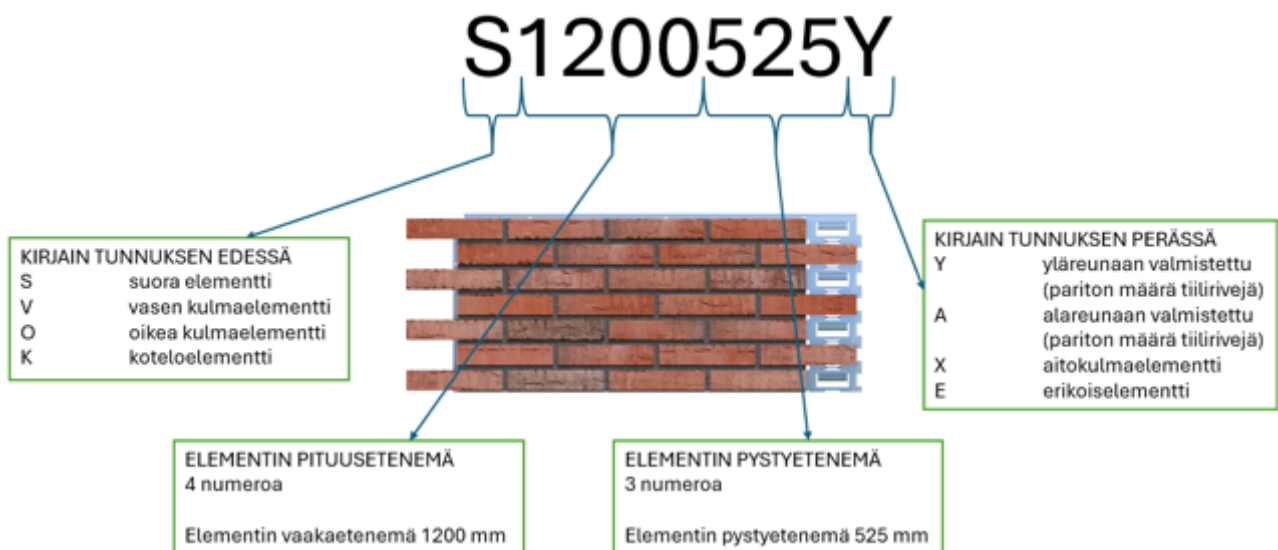
Kuva 3: Tiiliverhouslevyjen tunnukset
