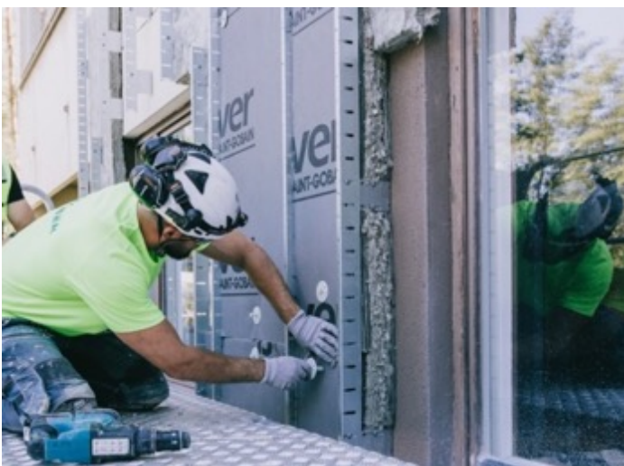
Kuva 32: Tuulensuojaeristyksen asentaminen
